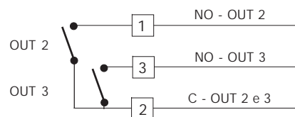
Fig. 8 COLLEGAMENTO DELLE USCITE A RELE'
