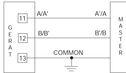
Abb.11 -ANSCHLUSS DER SCHNITTSTELLE RS-485
