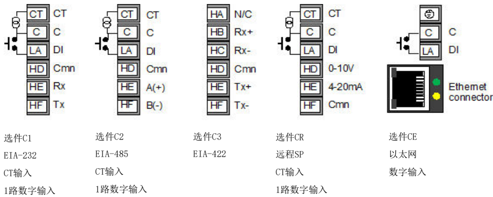
接线图中的助记符号
