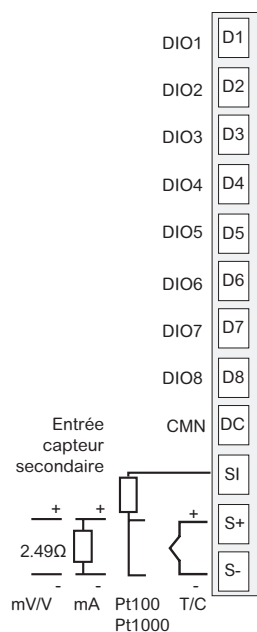
ENTRÉE PV 8 x ENTRÉES / SORTIES LOGIQUES
