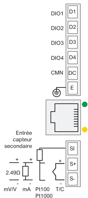
ENTRÉE PV ETHERNET 4 x ENTRÉES / SORTIES LOGIQUES
